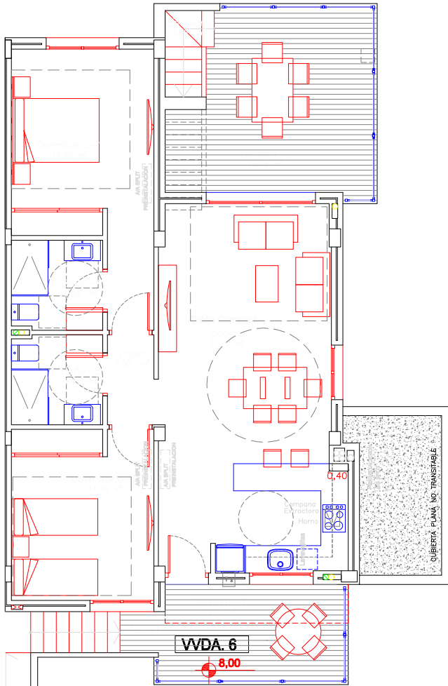
PLANTA PRIMERA.
